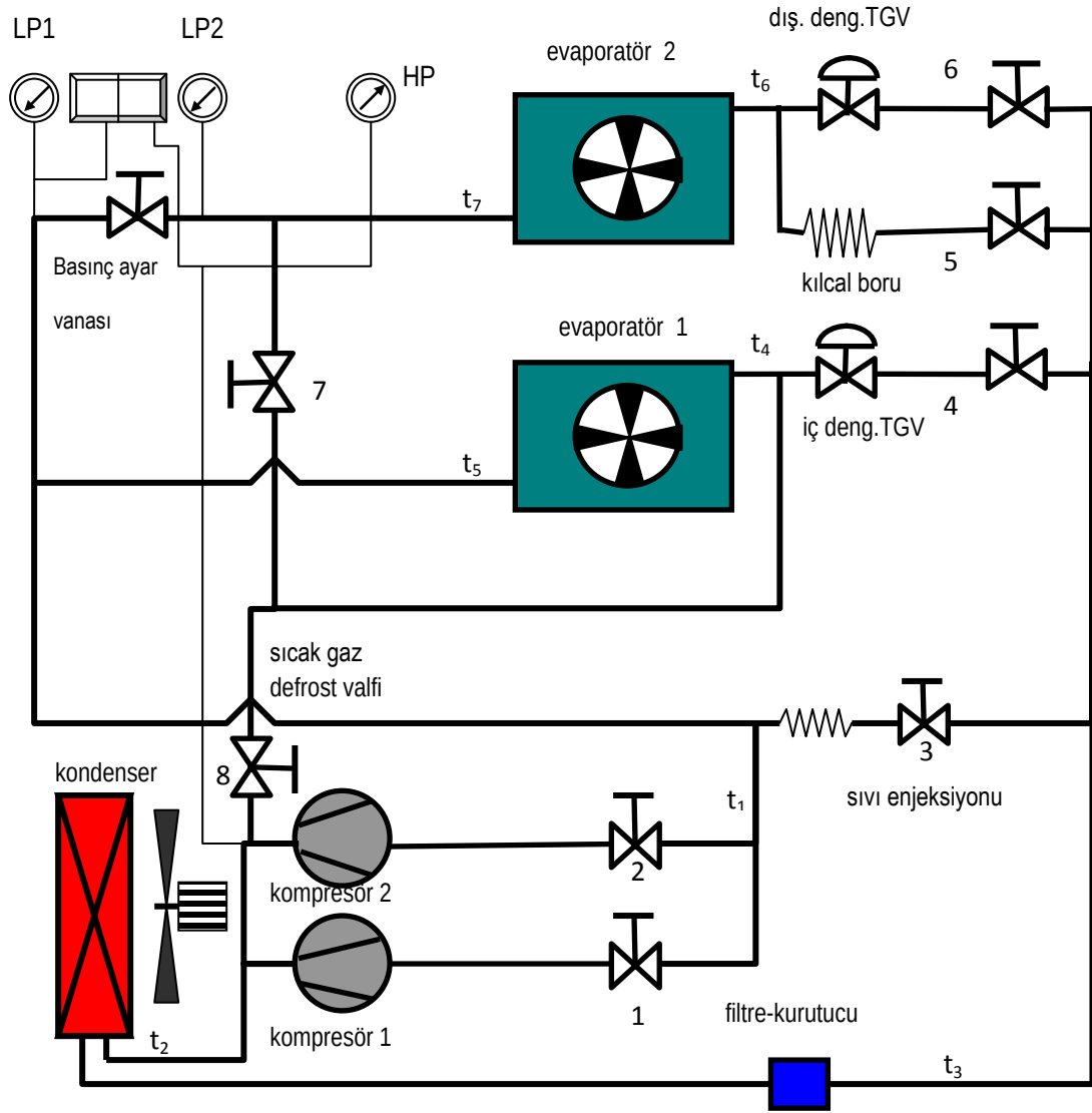
Şekil 2. Deney düzeneğinin şematik gösterimi.
