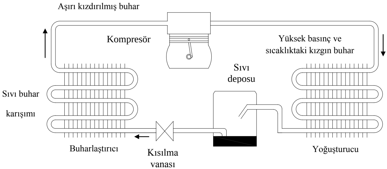
Şekil 1. Buhar sıkıştırmalı mekanik soğutma çevrimi.
