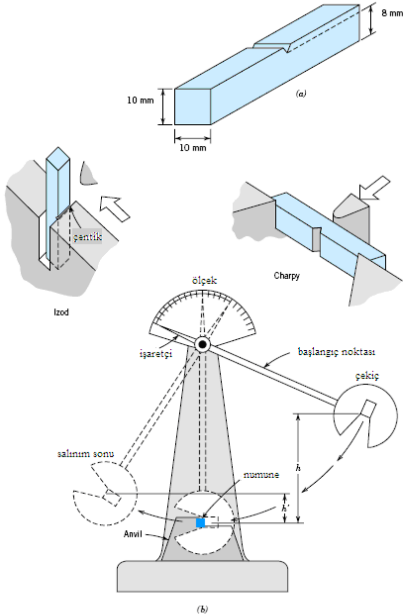
Şekil 2. Charpy ve Izod deneylerinde kullanılan deney numunelerinin çenelere yerleştirilmesi ve hesaplarda kullanılan ilgili parametreler.
