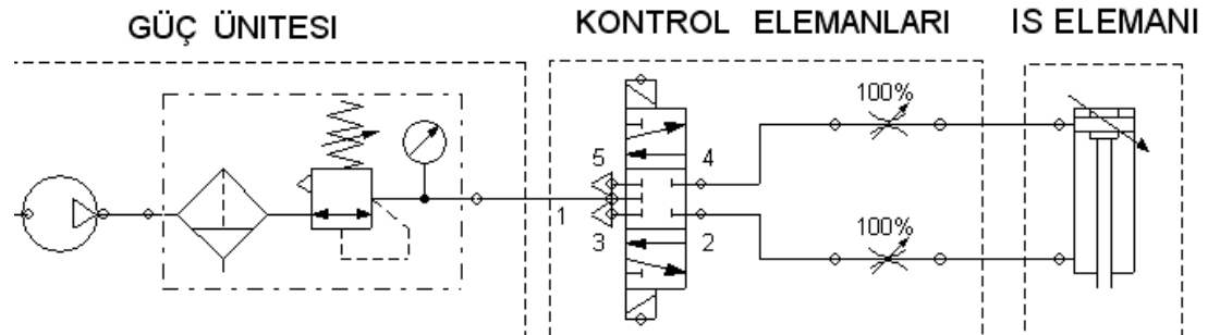
Şekil 2. Pnömatik Sistem
